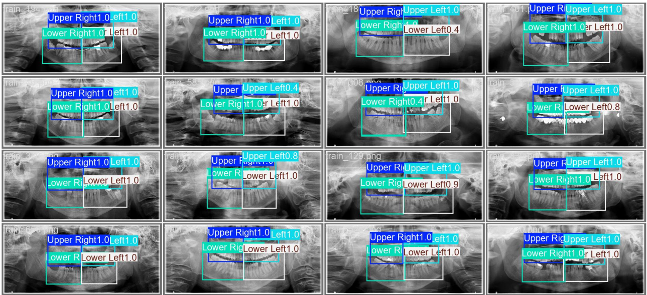
val_batch0_pred.jpg
