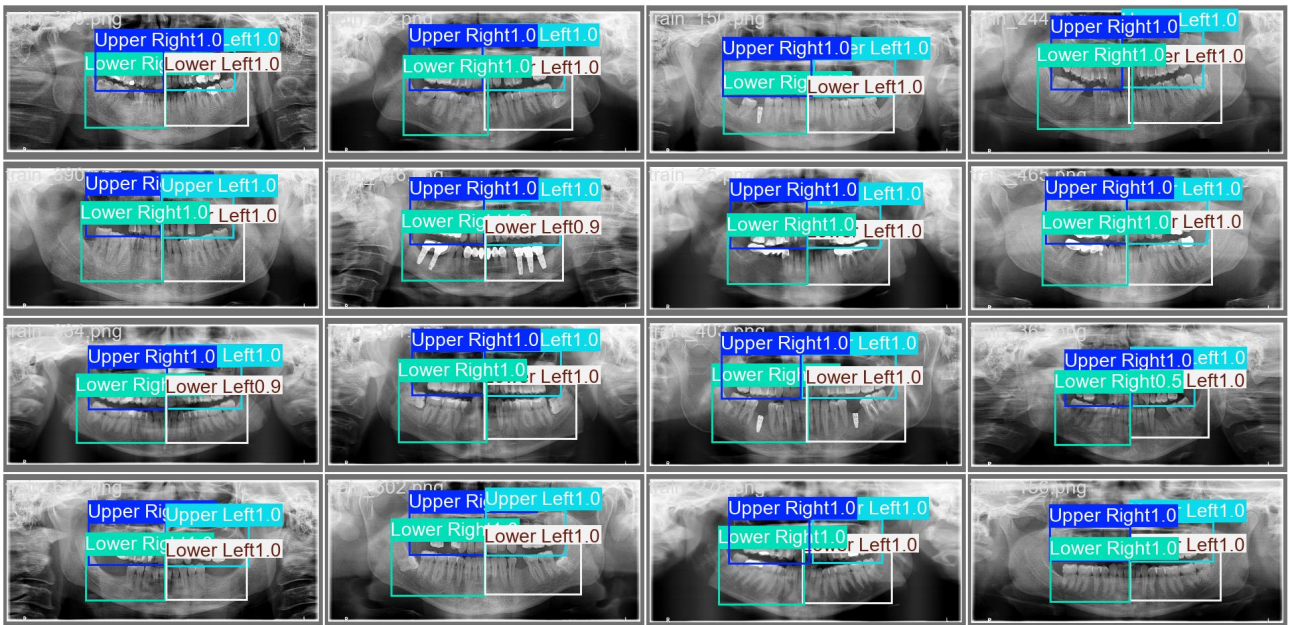
val_batch1_pred.jpg
